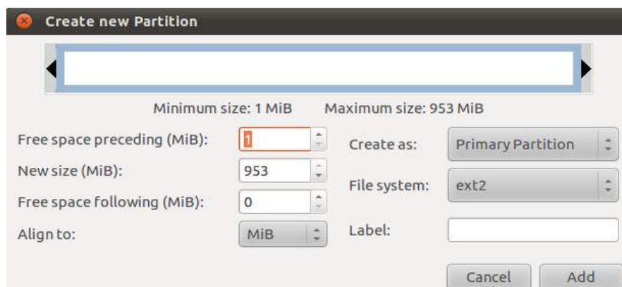
Slika 14.2.1.10 Primer pravljenja potrebnih particija za dva operativna sistema, korak 2
