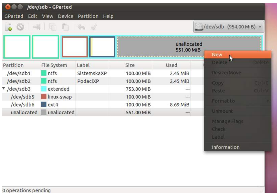
Slika 14.2.1.41 Primer pravljenja potrebnih particija za dva operativna sistema, korak 33
