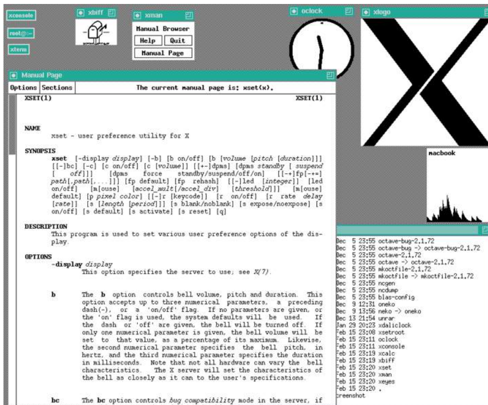
Slika 9.1 Izgled Juniks (engl. Unix) Radne površi (engl. Desktop) sa pokrenutim X Window System grafičkim korisničkim interfejsom ranih 1990-tih godina
