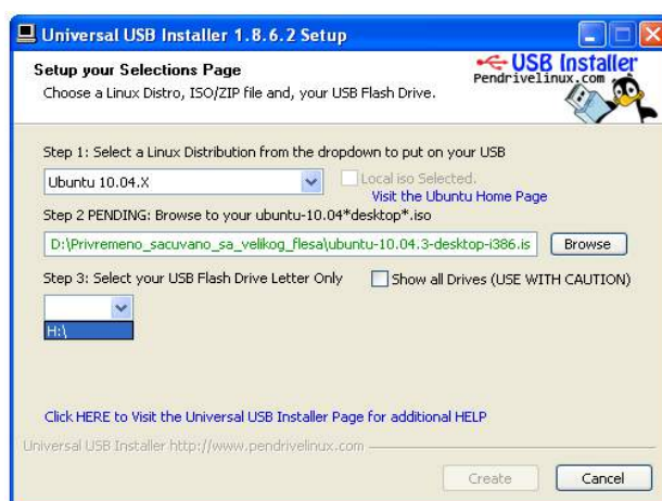
Slika 12.2.3.2.7 Pravljenje butabilnog USB-a, korak 7
