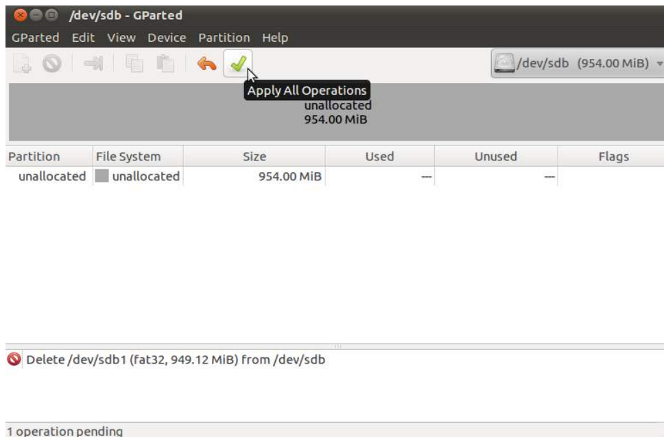
Slika 14.2.1.5 Proces brisanja željene particije, korak 2
