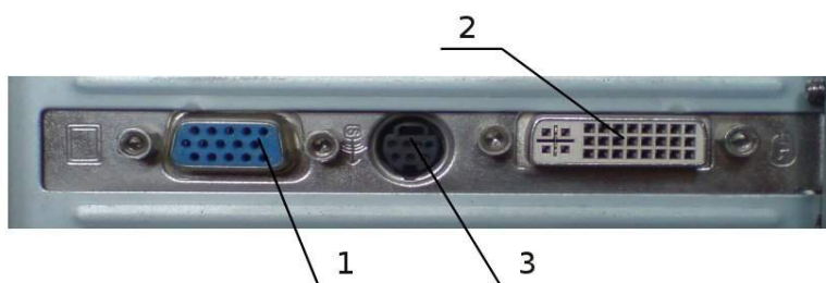
Slika 7.4.2 Priključci grafičke kartice na zadnjoj strani kućišta računara, ženski VGA priključak (1) i ženski DVI priključak (2), i tv izlaz (3)
